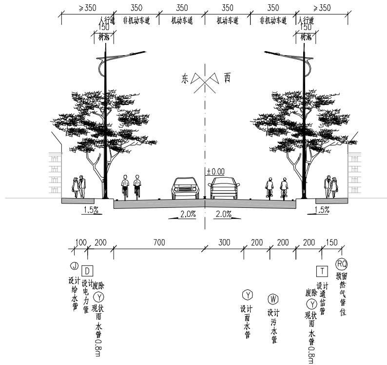
管综标准横断面图
