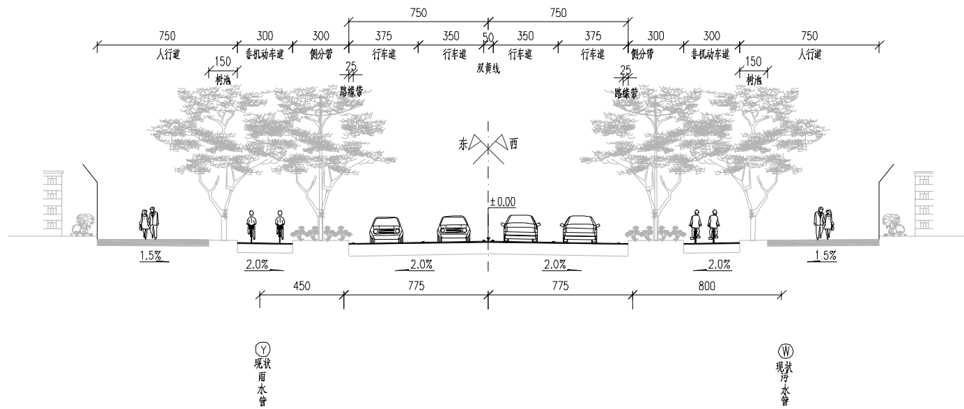
管综标准横断面图 (金家路)
